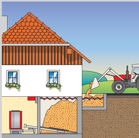
Hackgutlager im Keller des Wohnhauses mit waagrechter Befüllschnecke.
