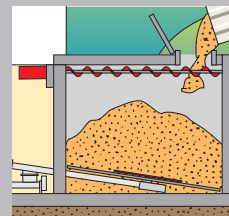
Optimale Hackgutverteilung in einem Erdbunker.
